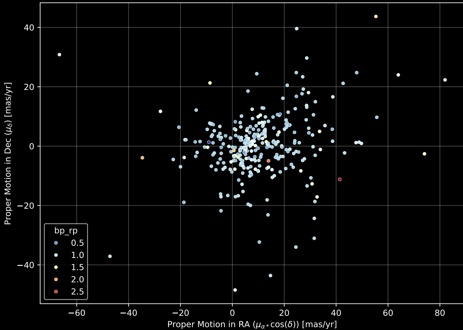
GALAH DR4 Field: [132] Proper Motion Diagram (n= 300)
