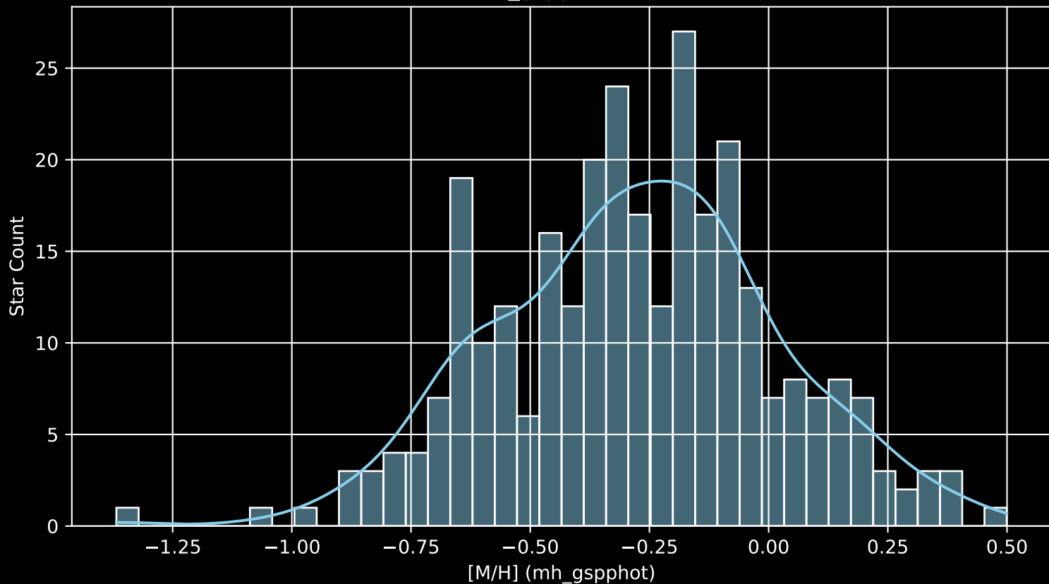
GALAH DR4 Field: [132] [M/H] (mh_gspphot) (n= 299)
