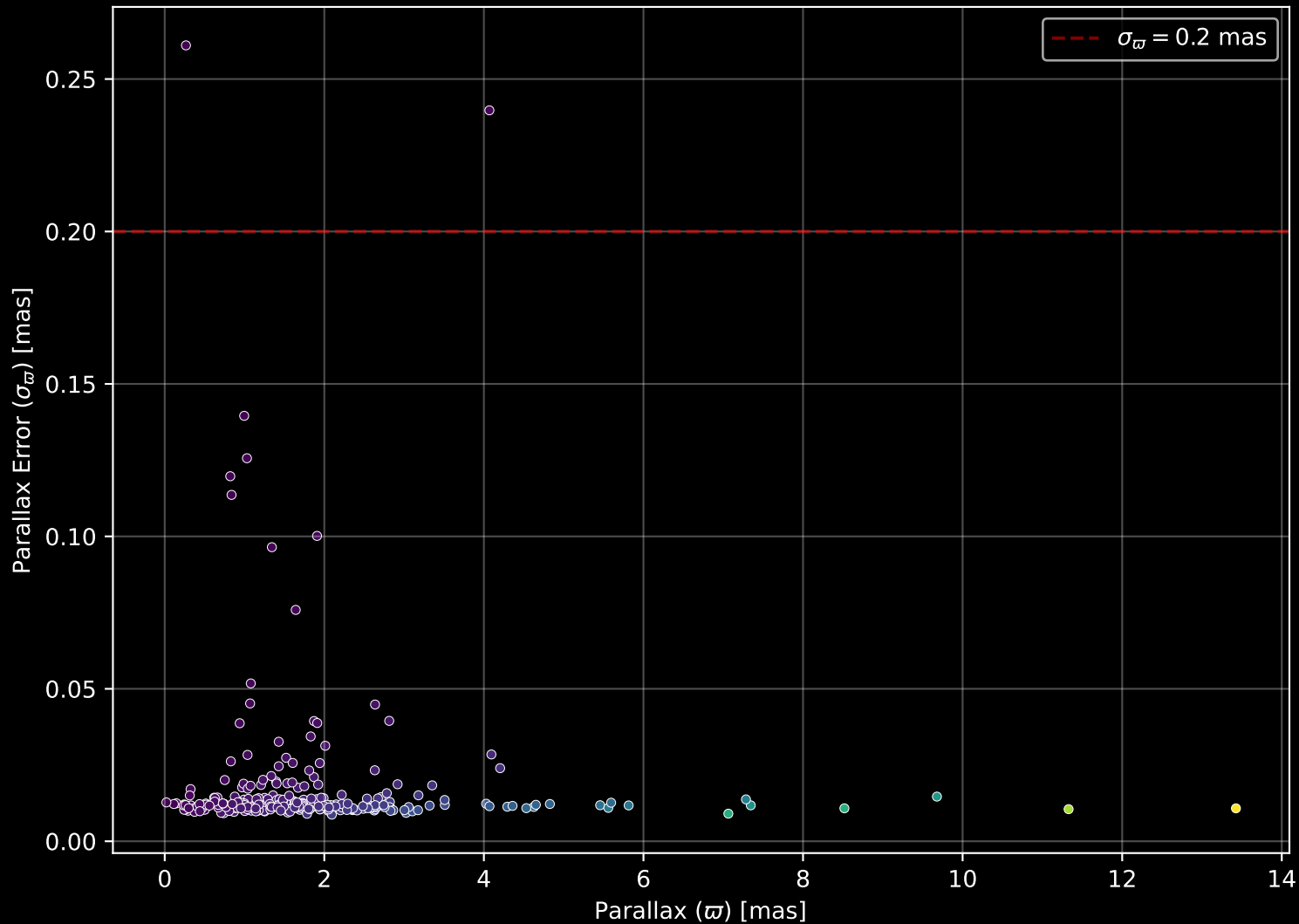
GALAH DR4 Field: [132] Parallax Quality (n= 300)
