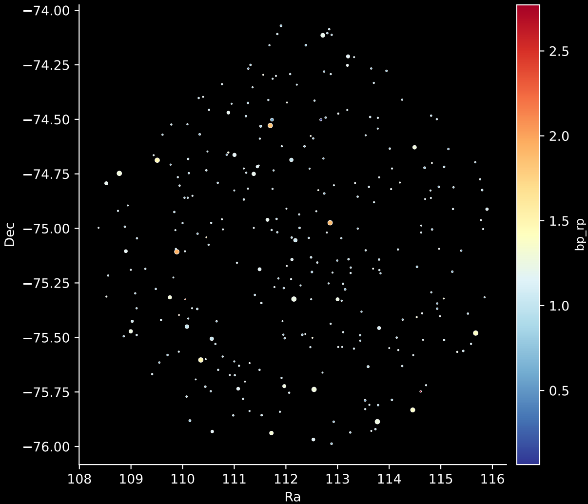
GALAH DR4 Field: [132] Stars: 300
