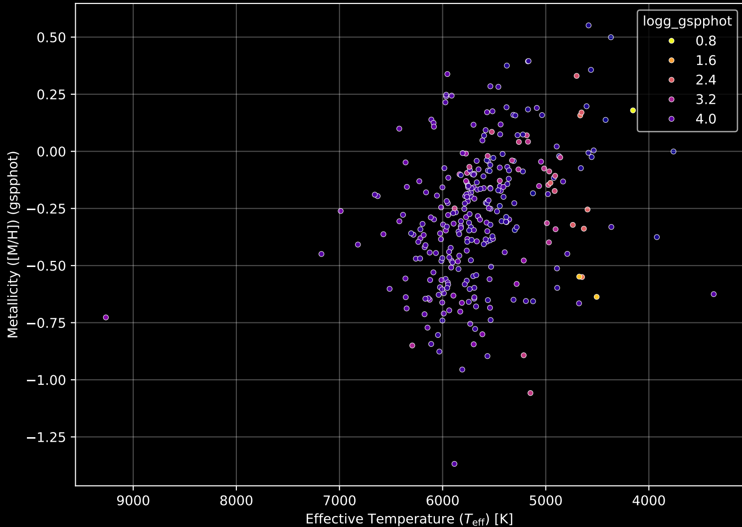
GALAH DR4 Field: [132] Stellar Population Parameters (n= 300)
